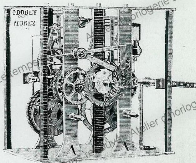
HORLOGE VERTICALE A SONNERIE
