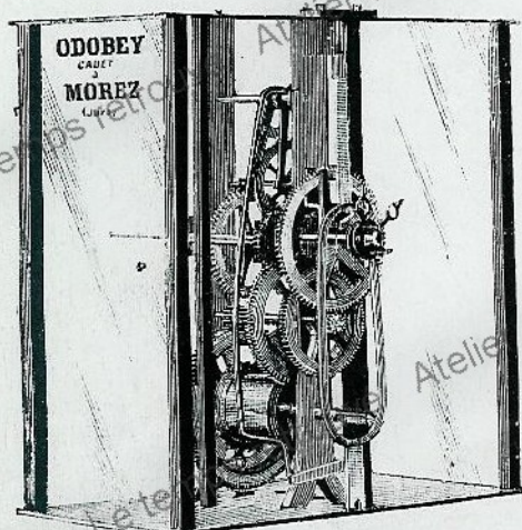
HORLOGE VERTICALE SANS SONNERIE
